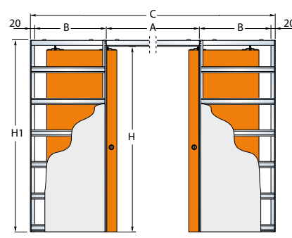
dvoukřídlé dveře / dvojkřídlové dvere
