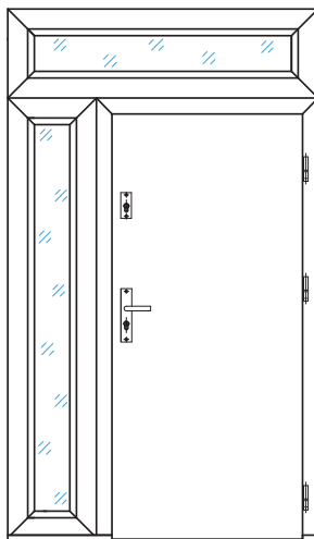
Dveře Disting s horním světlíkem a jedním bočním přístavkem
