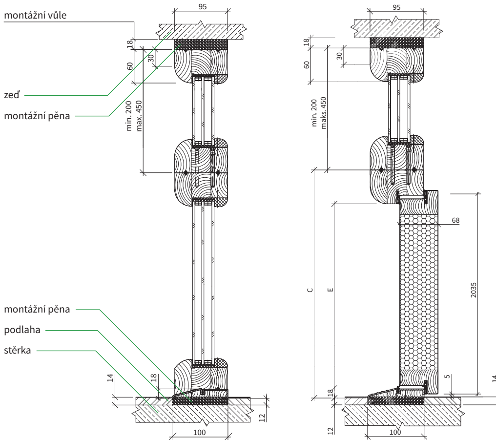
Průřez přes boční přístavek
